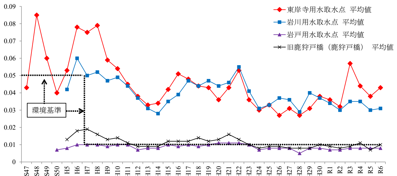
図3 岩戸川水系測定地点における砒素の経年変化（単位:mg/L）
