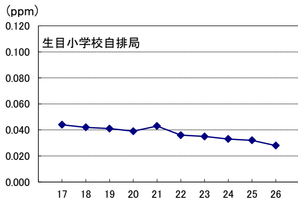
光化学オキシダント(昼間の日最高1時間値の年平均値)
